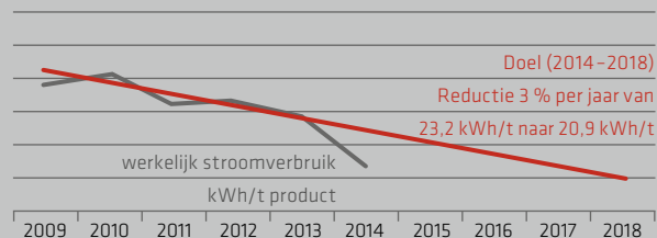
Stroomverbruik in kWh per t geproduceerd product
