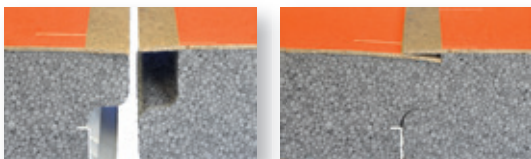
Gepatenteerde randafwerking voor types t/m 5.0
