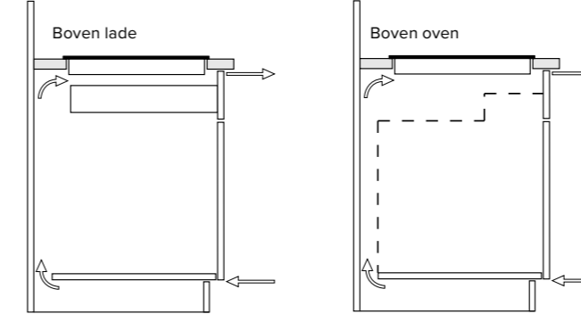
Inbouwtekening inductiekookplaat
